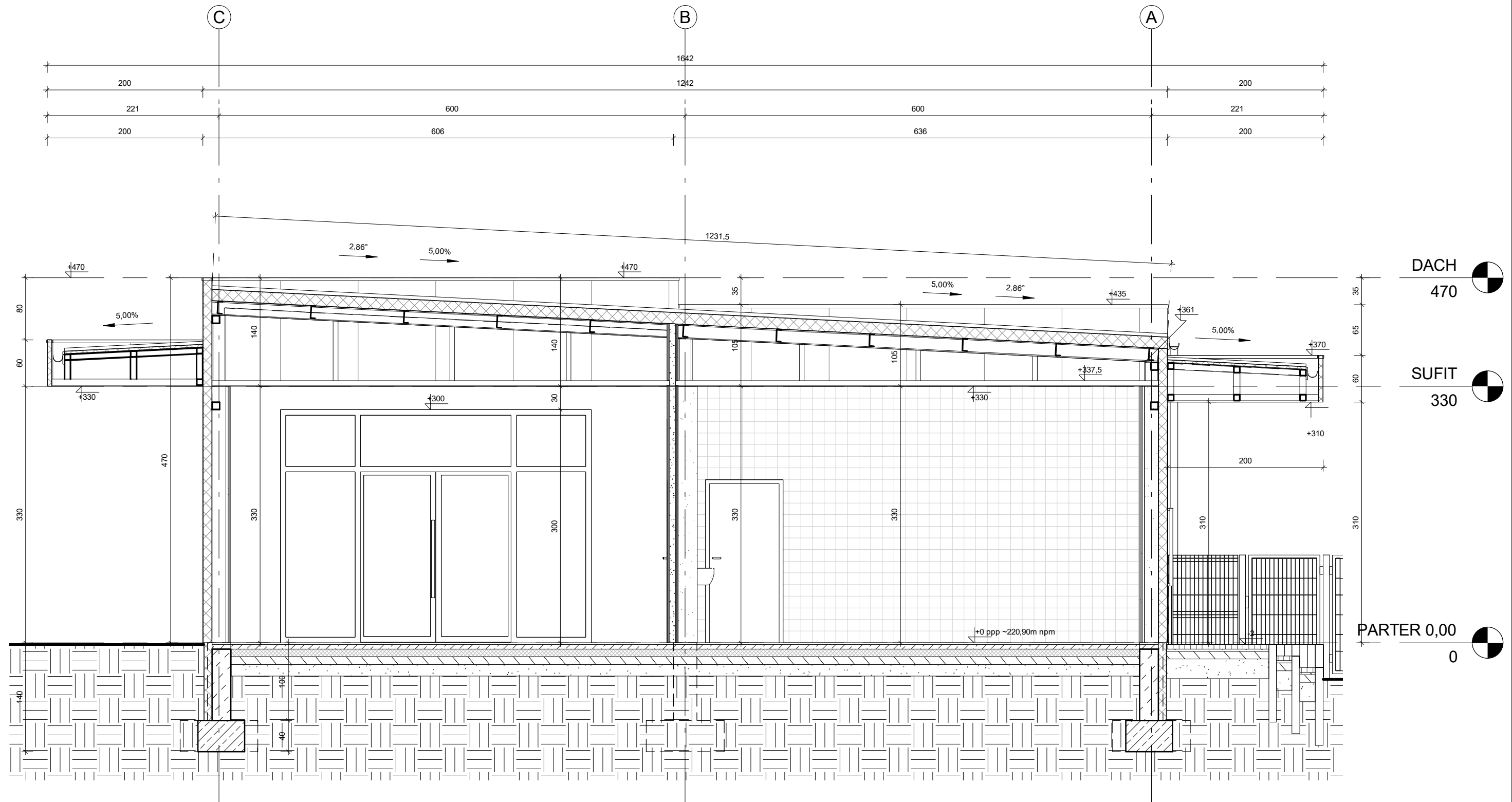
1 PRZEKRÓJ A-A 1 : 50
