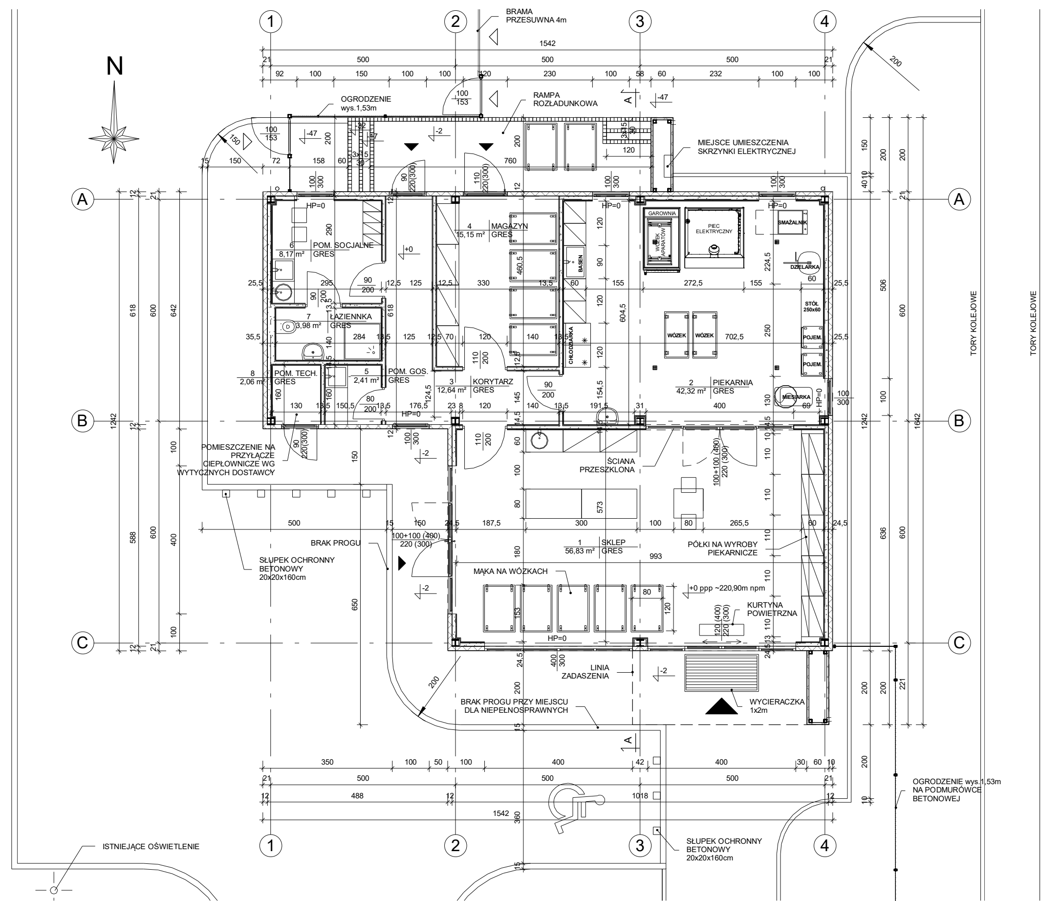
1 PARTER 0,00 1 : 100
